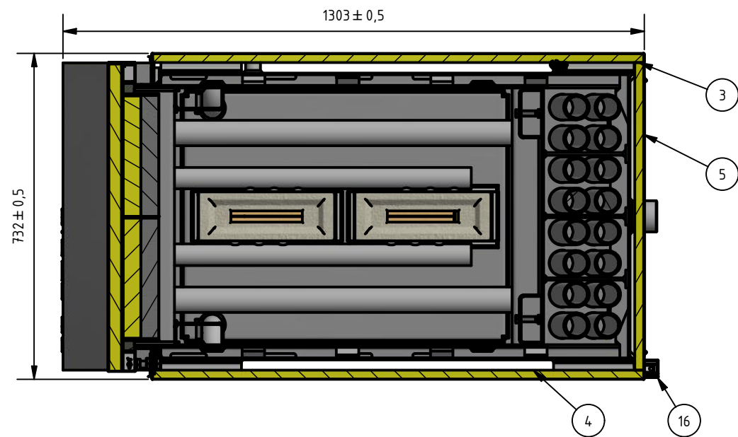
C-C ( 1 : 12 )
